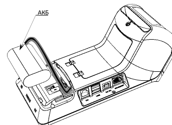
Рисунок 3. Установка аккумулятора
